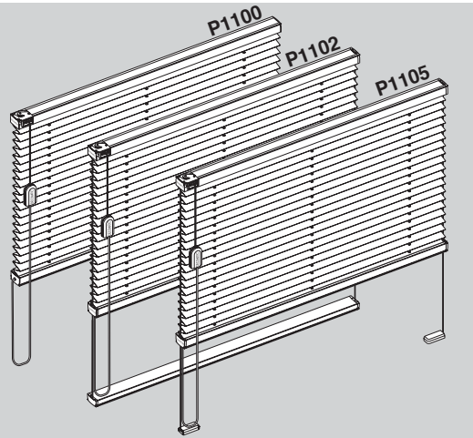
P1100 – volně zavěšené plisé – šňůrové ovládání P1102 – včetně vedení lanky v dolním profilu P1105 – včetně vedení lanky v držácích
