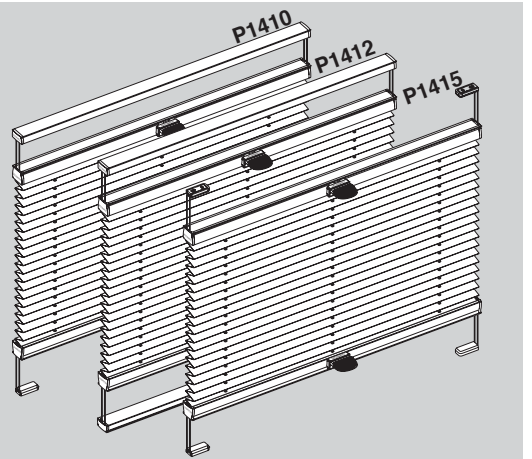
P1410 – napínané plisé s úchytem, variabilním svazkem a napínáním vodících šňůr v dolním a horním napínacím profilu P1412 – včetně šňůrového vedení/napínací profil P1415 – včetně šňůrového vedení/napínací držák
