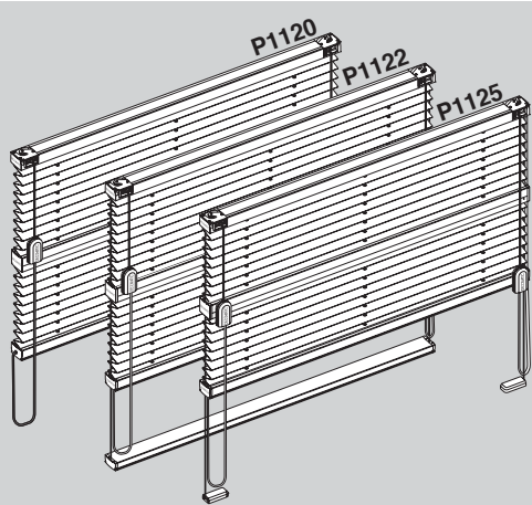
P1120 – volně zavěšené plisé se dvěma ovládacími jednotkami a dvěma svazky P1122 – včetně vedení provlečené v profilu P1125 – včetně vedení/napínací držáky
