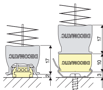
Zesílený profil 17 mm
