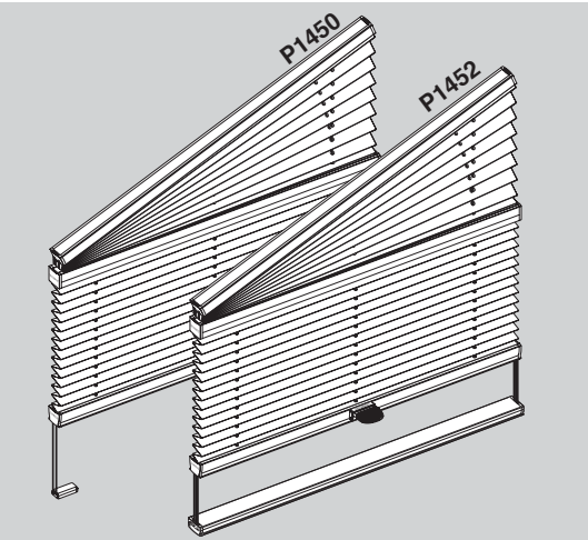
P1450 – napínané sešíkmené plisé s úchytem a napínanou šňůrou/napínací držák P1452 – včetně šňůrového vedení/napínací profil
