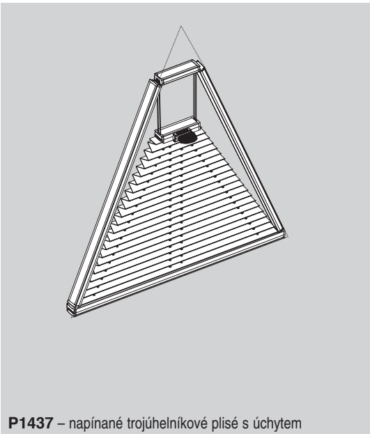
P1437 – napínané trojúhelníkové plisé s úchytem
