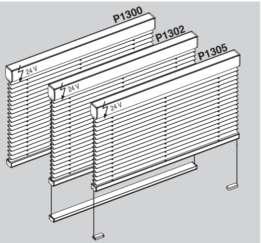
P1300 – volně zavěšené plisé s motorovým ovládáním P1302 – včetně šňůrového vedení/napínací profil P1305 – včetně šňůrového vedení/napínací držák
