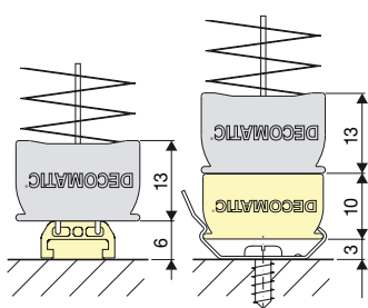
Standardní profil 13 mm
