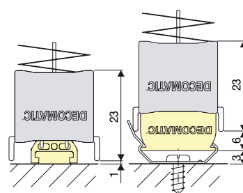
Zesílený profil 23 mm
