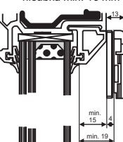
Trojité zasklení 1 distanční podložka hloubka min. 15 mm
