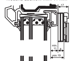
Trojité zasklení 2 páry distančních podložek hloubka zasklení min. 11 mm
