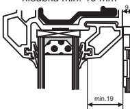
Dvojitě zasklení bez distančních podložek hloubka min. 19 mm
