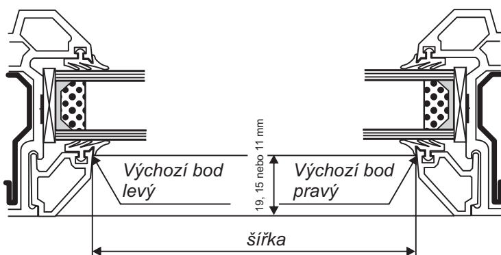
Trojité zasklení 1 distanční podložka hloubka min. 15 mm
