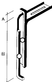
Držák krycího plechu
