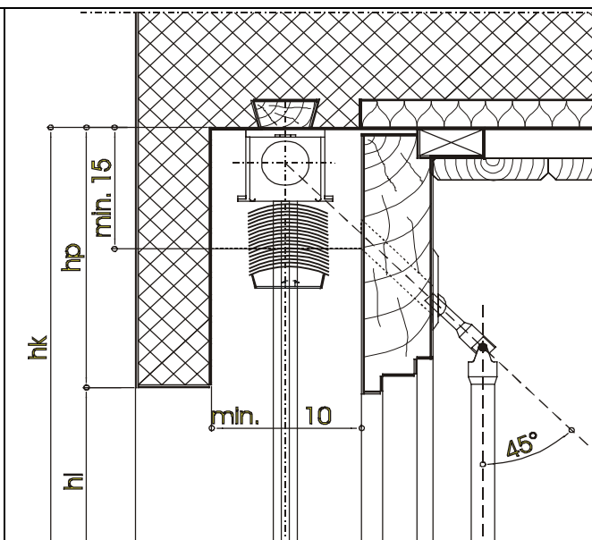
EXT 50 mm - vertikální řez- montáž do stavební dutiny
