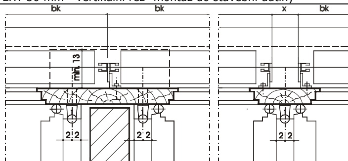
EXT 50 mm - vertikální řez- montáž do stavební dutiny
