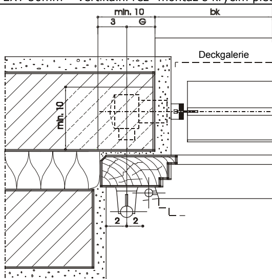
EXT 50 mm - horizontální řez - montáž do ostění
