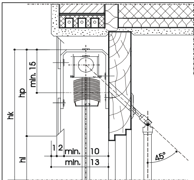
EXT 50mm – vertikální řez- montáž s krycím plechem
