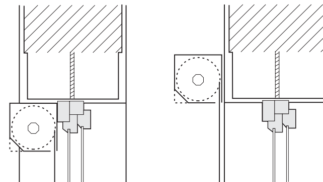
PŘÍKLADY MONTÁŽE
